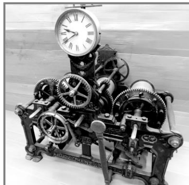
Rekonstruovaný hodinový stroj
