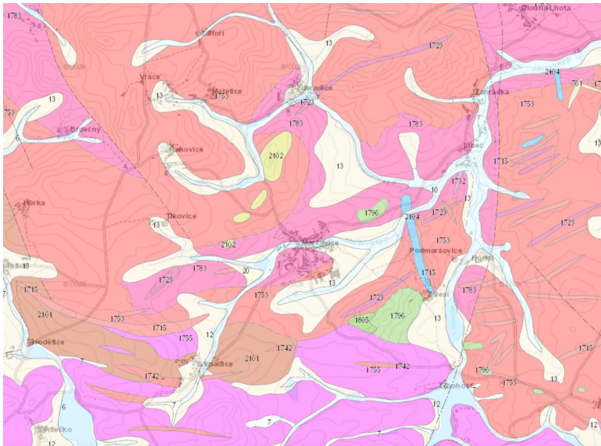
Mapa 1 Geologická mapa území (Zdroj: Česká geologická služba)
