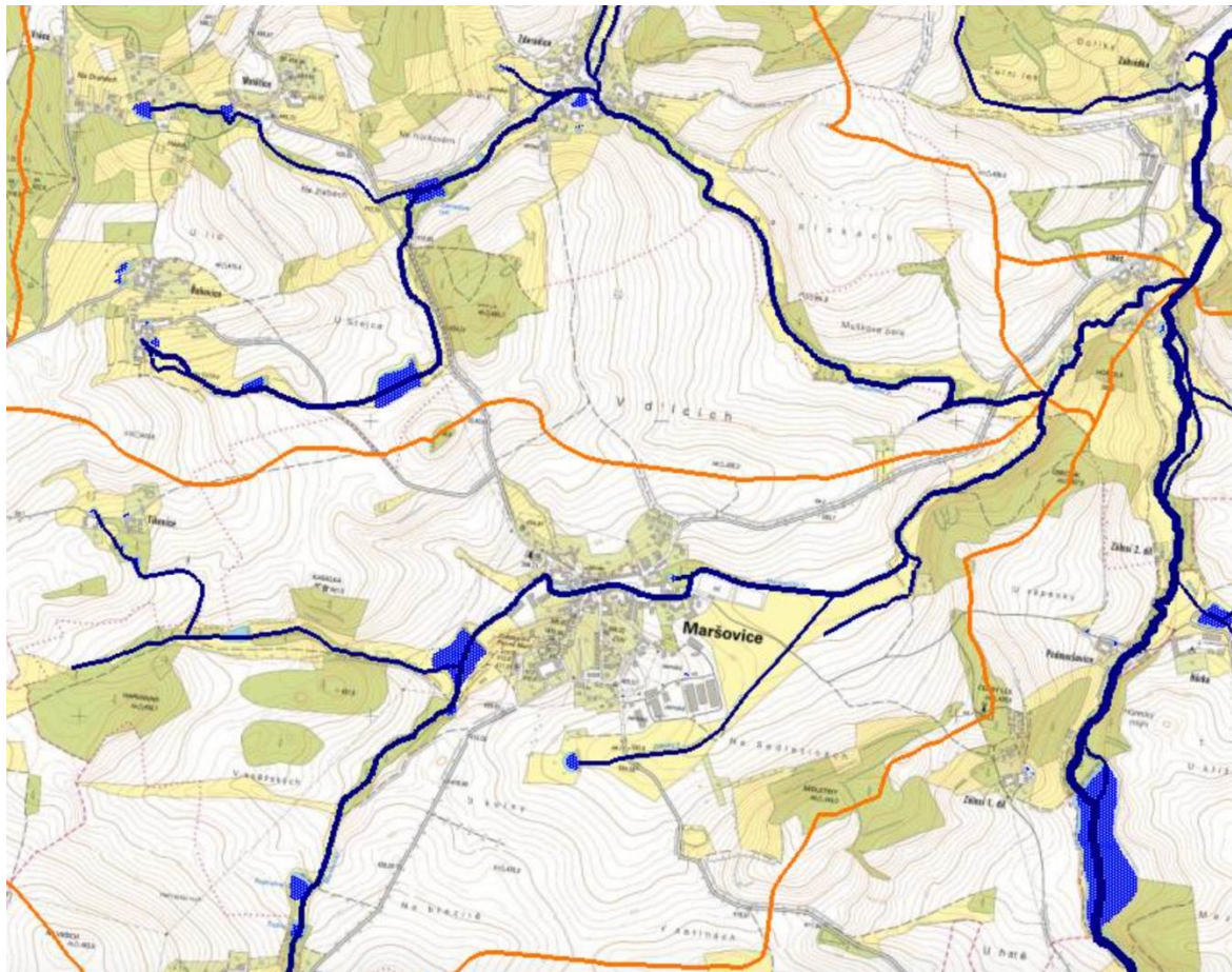
Mapa 2 Hranice hydrologického povodí 3. řádu (oranžové linie), vodní toky a vodní nádrže
